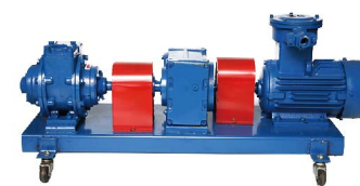
减速机结构 Coupling Drive
